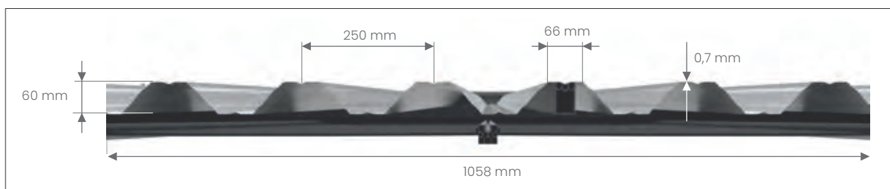
Vue de coupe de la tôle a plis en trapèze T60P (mm) | Sezione trasversale della lamiera trapezoidale T60P (mm)
