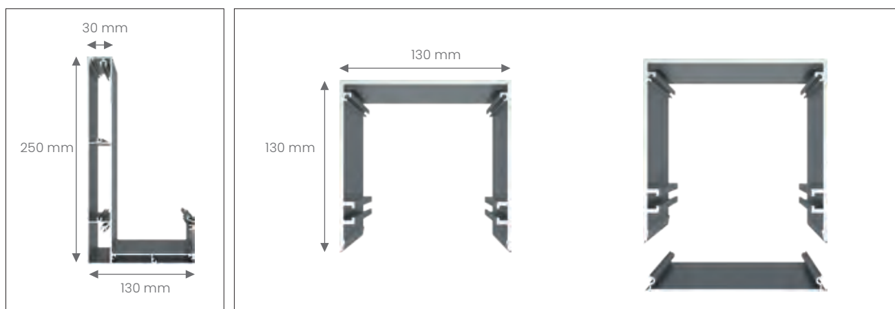
Profilé de construction
